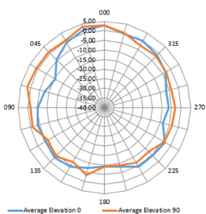
Elevationsebene (Seitenansicht)
