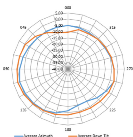
Azimutebene (Draufsicht)
