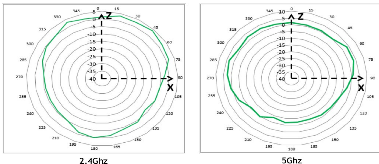
图1 OmniAccess AP1321 天线模式图
