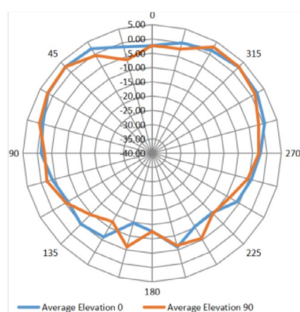
仰角平面（侧视图）
