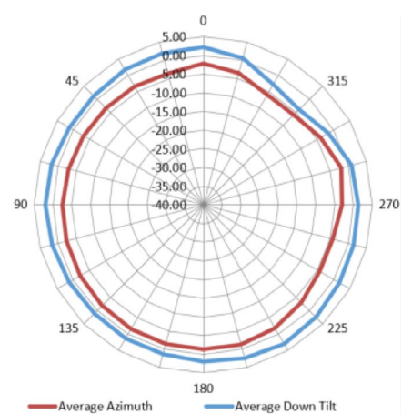
方位平面（顶视图）
