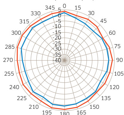
Azimet-Ebene (Draufsicht) - 2,45 GHz
