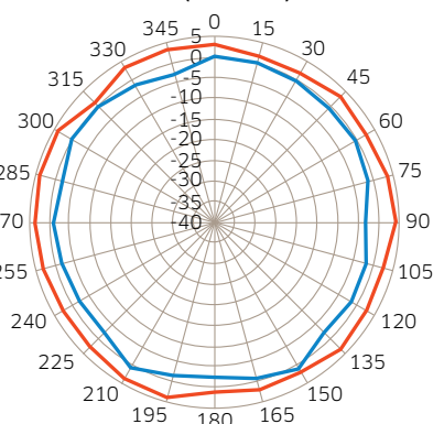
Azimet-Ebene (Draufsicht) - 5 GHz L
