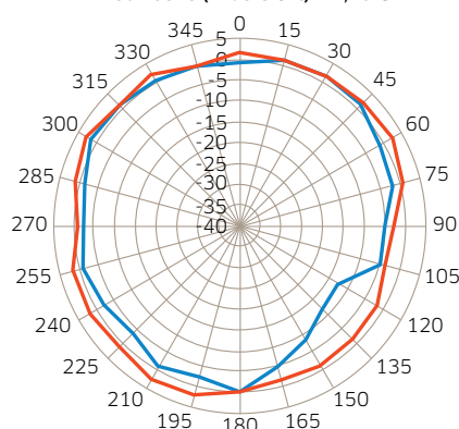
Azimet-Ebene (Draufsicht) - 2,45 GHz
