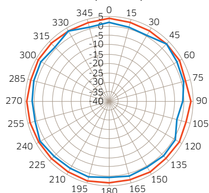
Azimet-Ebene (Draufsicht) - 5 GHz H
