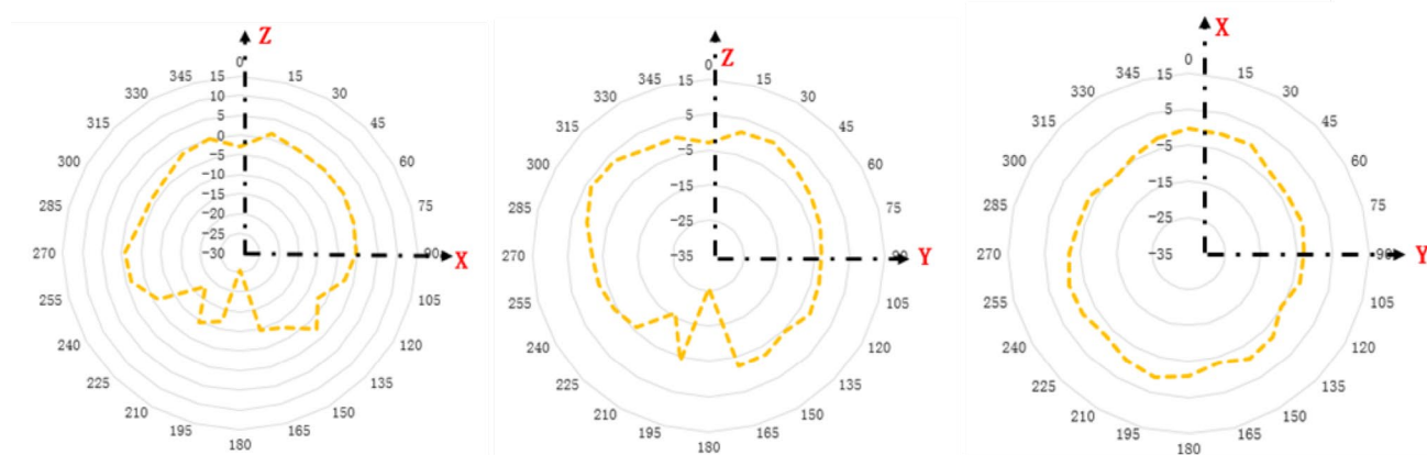
图3: BLE 辐射模式图
