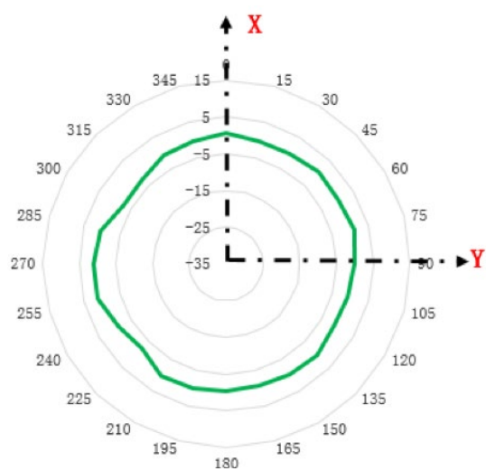
图1: OmniAccess AP1361天线模式图
