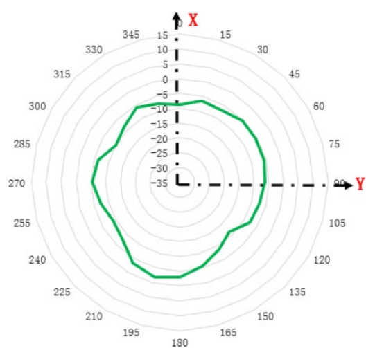
图2: OmniAccess AP1361D天线模式图
