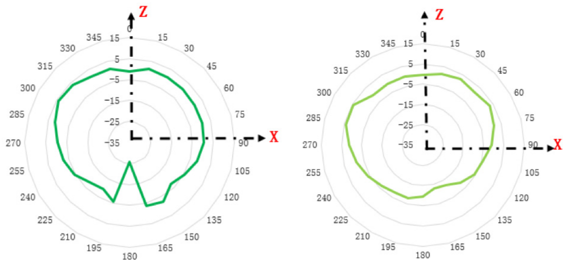
Ansichtsebene (Seitenansicht, Winkel von 90 Grad)
