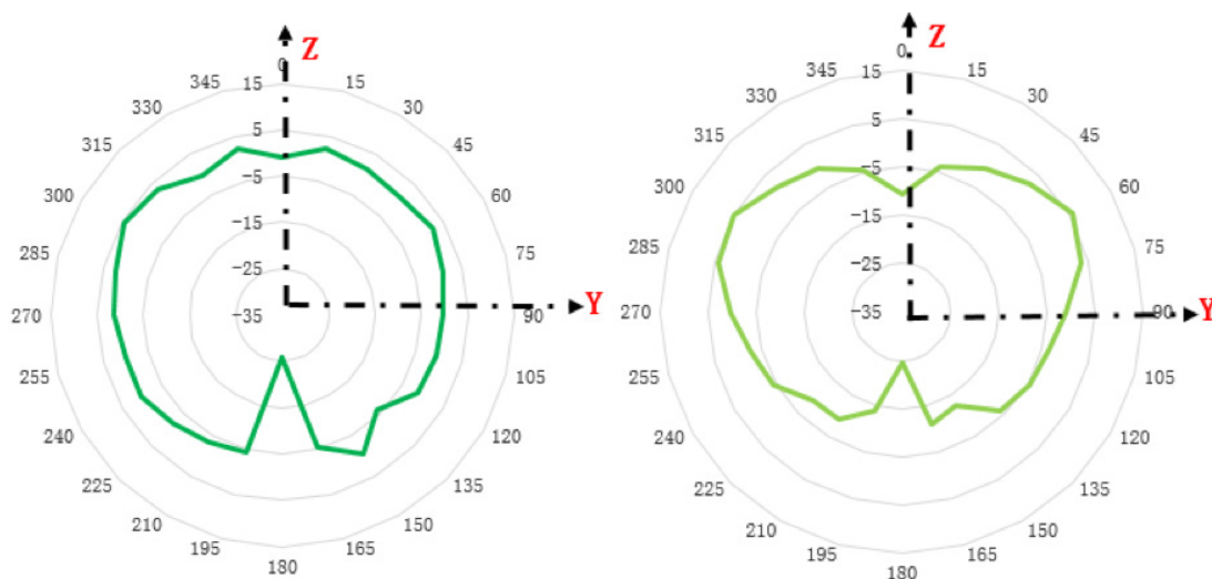
Ansichtsebene (Seitenansicht, Winkel von 90 Grad)
