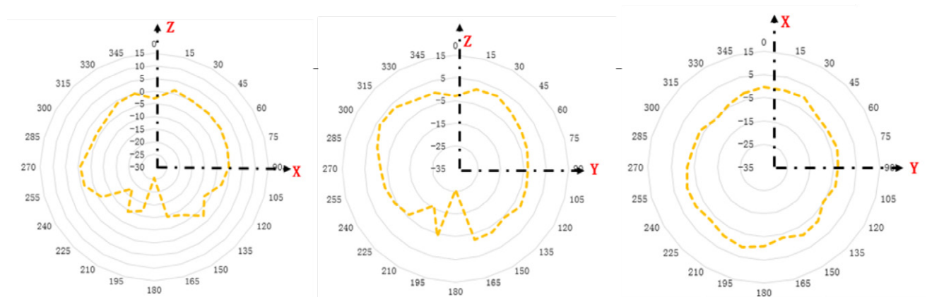
Abbildung 3: BLE-Abstrahlmuster
