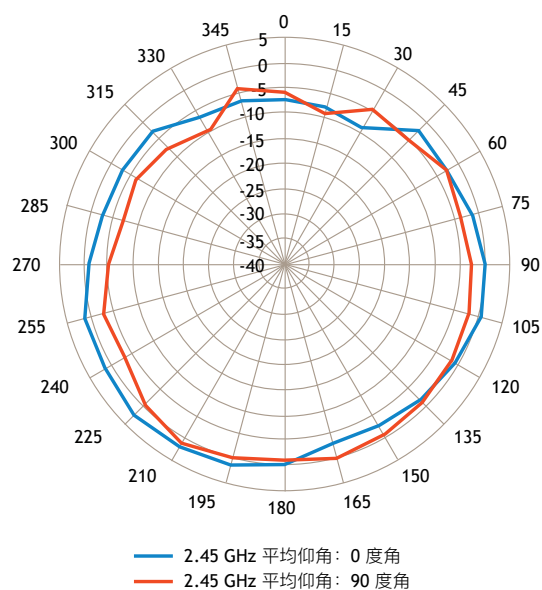
仰角平面 (侧视图) - BLE
