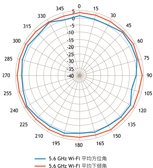
方位平面 (顶视图) - 6 GHz
