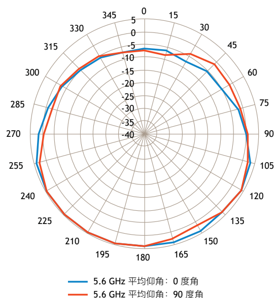
仰角平面 (侧视图) - 6 GHz
