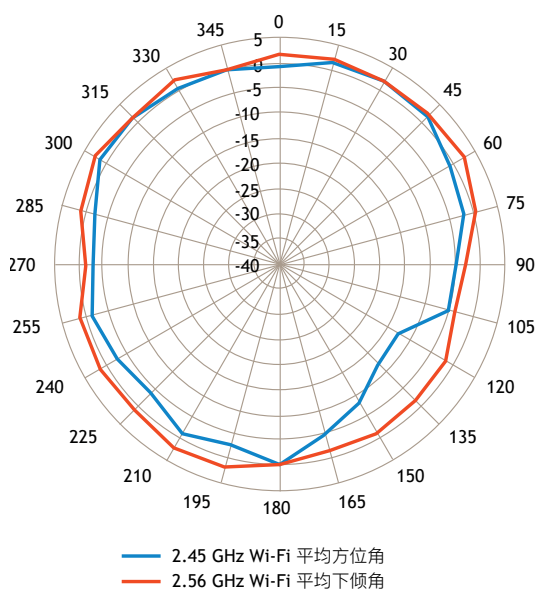
方位平面 (顶视图) - BLE
