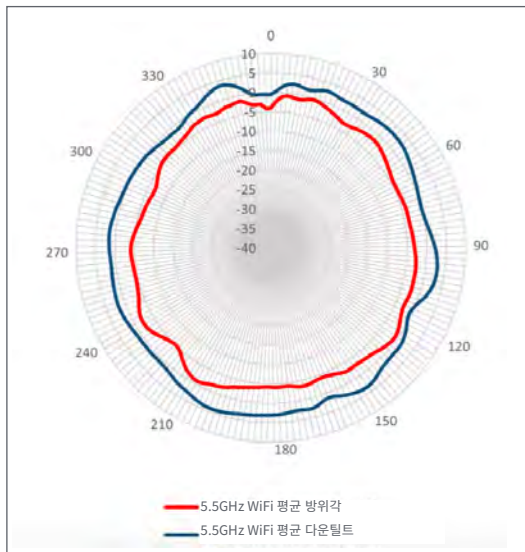
고도면(측면도) - 5GHz
