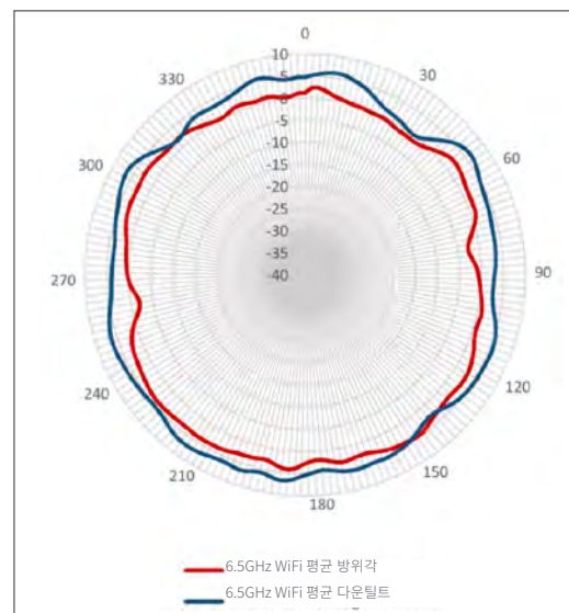
고도면(측면도) - 6GHz
