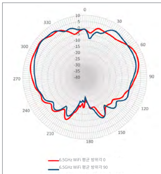
방위면(평면도) - 6GHz
